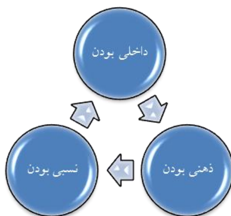
شکل ۲. مؤلفه‌های امنیت
